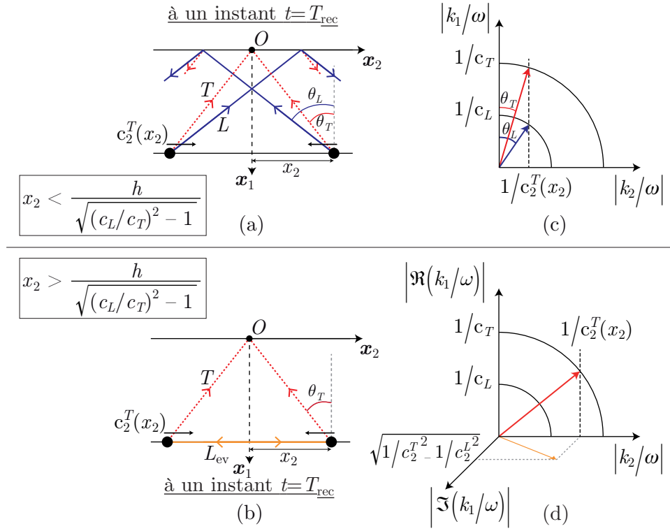
Fig. 6.4 – Illustrations des ondes générées par deux sources en mouvement à la vitesse \pm c_2^T(x_2) au point de mesure d'abscisse x_2 : (a) dans le cas |x_2| < h/\sqrt{(c_L/c_T)^2 - 1} et (b) dans le cas opposé. (c)-(d) Diagrammes des lenteurs de phases pour un matériau isotrope associé respectivement aux cas (a) et (b). Les traits pointillés verticaux représentent dans les deux cas la lenteur des sources en mouvement.
